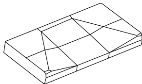
ПАНДУС ВЪЕЗДНОЙ 3000 (4000–6000) × 1500 × 300 (150)
