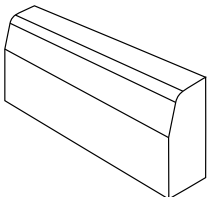
БОРДЮР МОСТОВОЙ 1000 × 450 × 180 мм 1000 × 600 × 180 мм 1000 × 600 × 150 мм с фаской
