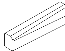
БОРТОВОЙ КАМЕНЬ ДОРОЖНЫЙ ПРАВЫЙ 1000 × 300 / 220 × 150 мм
