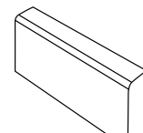
КАМЕНЬ САДОВЫЙ 500 × 200 × 50 мм
