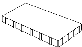
ПЛИТА 600 × 400 × 60 мм 600 × 400 × 80 мм 800 × 400 × 80 мм 800 × 400 × 100 мм
