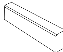
ДОРОЖНЫЙ БОРДЮРНЫЙ КАМЕНЬ 1000 × 300 × 150 мм с фаской 1000 × 300 × 150 мм с двумя фасками
