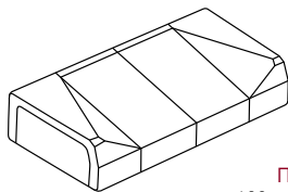
СТЕНОВОЙ ДВУХПУСТОТЫЙ БЛОК 390 × 190 × 190 мм
