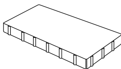
ПЛИТА 600 × 300 × 60 мм — без фаски 600 × 300 × 80 мм 600 × 300 × 100 мм
