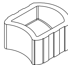
ПАРКФЛОР 500 × 430 × 250 мм 410 × 360 × 250 мм
