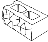
БЕТОННЫЙ КОЛОТЫЙ ПУСТОТЕЛЫЙ ДВУХСТОРОННИЙ БЛОК 390 × 190 × 190 мм
