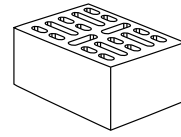
18-ЩЕЛЕВОЙ БЛОК 380 × 250 × 140 мм
