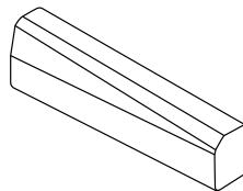
БОРТОВОЙ КАМЕНЬ ДОРОЖНЫЙ ЛЕВЫЙ 1000 × 300 / 220 × 150 мм
