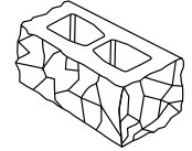
БЕТОННЫЙ КОЛОТЫЙ ПУСТОТЕЛЫЙ ТРЕХСТОРОННИЙ БЛОК 390 × 190 × 190 мм
