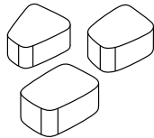
ВЕЕР 118 × 78 × 109 / 60 мм 118 × 46 × 146 / 60 мм 88 × 118 × 60 мм
