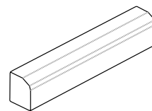
БОРТОВОЙ КАМЕНЬ ПОНИЖЕННЫЙ 1000 × 220 × 150 мм
