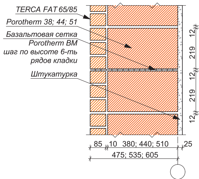
Стена тип 2
