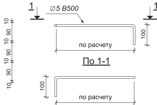
Анкер А-2
