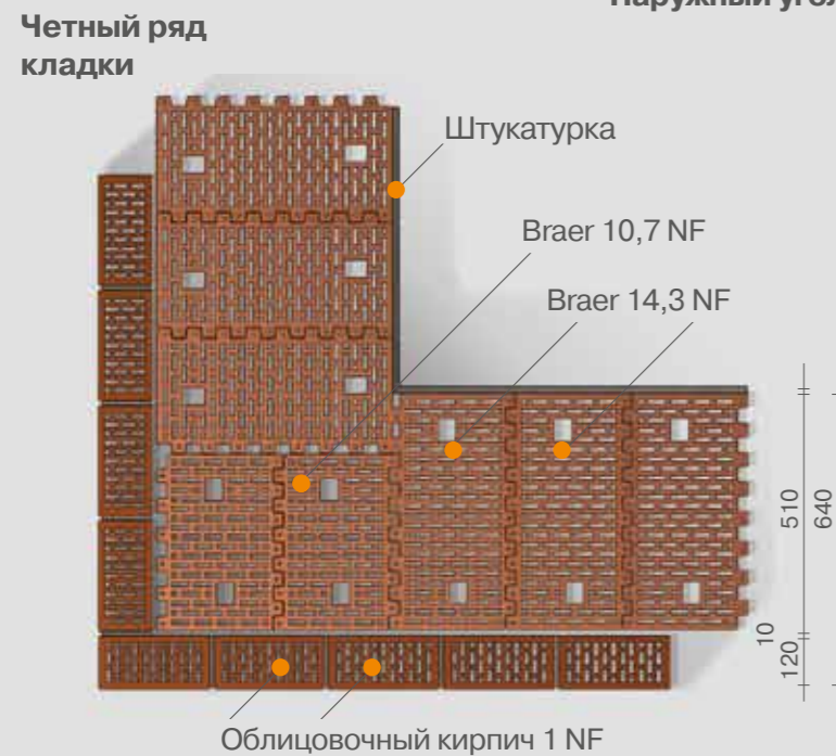
Четный ряд кладки Наружный угол стены
