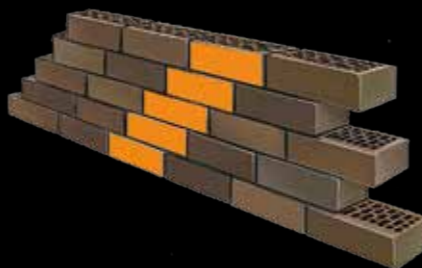
3 ЛОЖКОВАЯ КЛАДКА КОСОЕ СМЕЩЕНИЕ НА 1/4 КИРПИЧА
