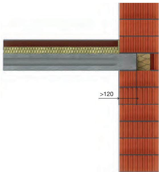
Рис. 13. Опирание плит перекрытия на кладку из блоков Porotherm
