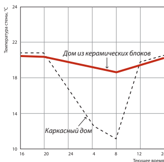
Рис. 8. Поддержание среднесуточной комнатной температуры при переключении работы отопления на пониженный режим
