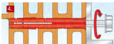
4. Заворачивание шурупа
