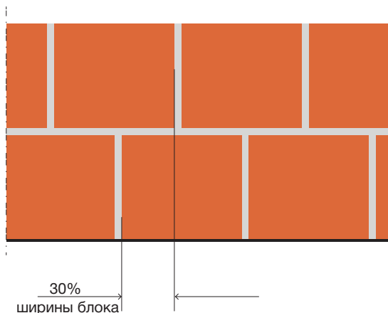
Рис. 9. Минимальная перевязка вертикальных швов
