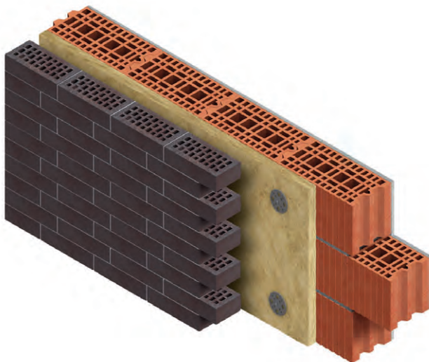
Рис. 4. Конструкция стены из блоков Porotherm 20, минераловатных плит и облицовочного кирпича
