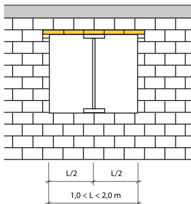
Схема установки подпорной стойки под перемычки длиной до 2,0 м
