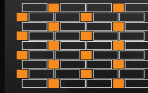
Цепная кладка
