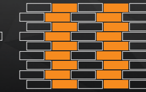
Ложковая кладка смещение на 1/4 кирпича
